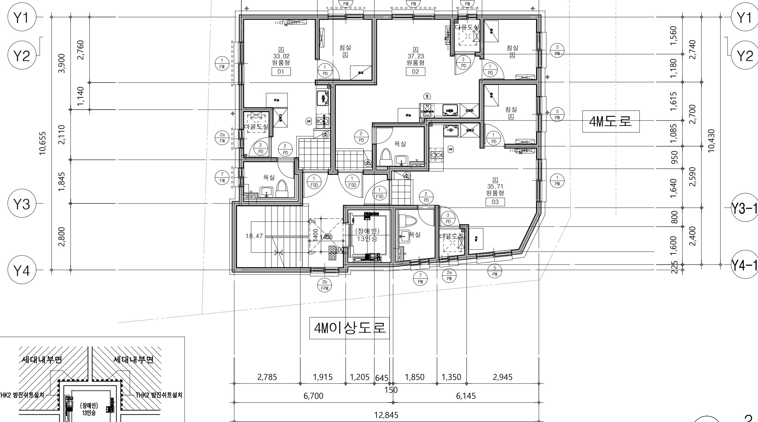
승강로에 면한 각층세대부분 방진셔틀설치도
