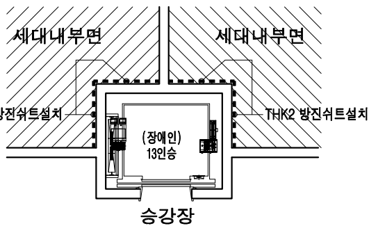
승강로에 면한 각층세대부분 방진셔틀설치도
